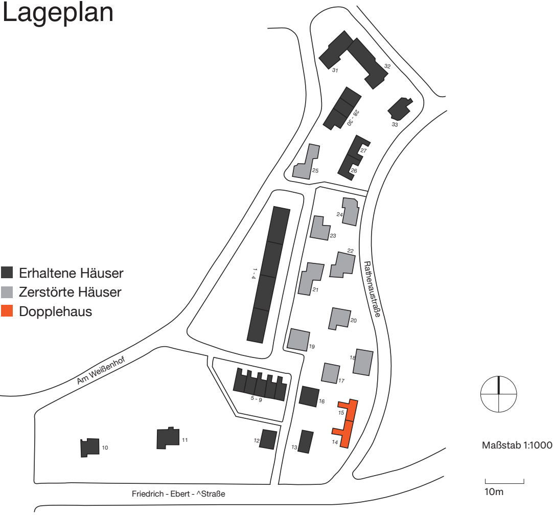
Lageplan
