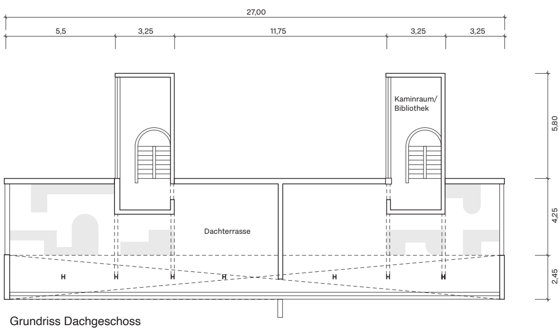
Grundrisse
