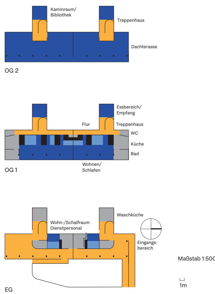
Gebäudenutzungs-schemata
